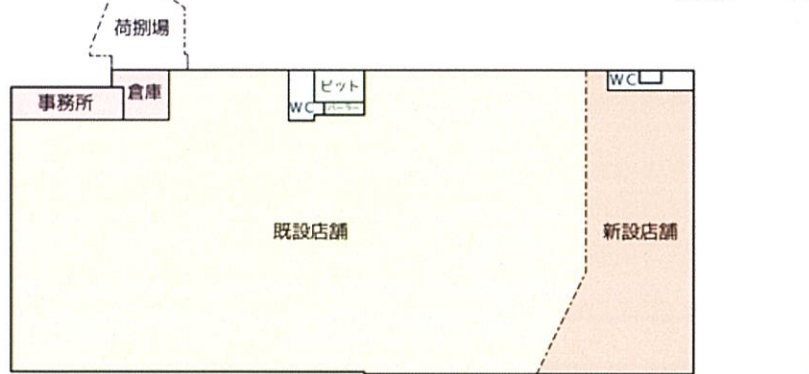
店舗平面図
